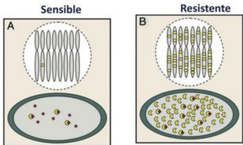
Figura 6. Resistencia al glifosato resultado de la amplificación génica. En una planta sensible (A), el número de copias del gen EPSP (de color amarillo en los cromosomas) produce enzima EPSPS en los cloroplastos que es inhibida por el herbicida glifosato (en rojo) provocando la muerte de la planta. En una planta resistente (B) con amplificación génica del enzima EPSPS presente en varios cromosomas, conlleva un incremento de enzima EPSPS y el glifosato no puede inhibir toda el enzima EPSPS disponible. Tomado de Powless (2010).
