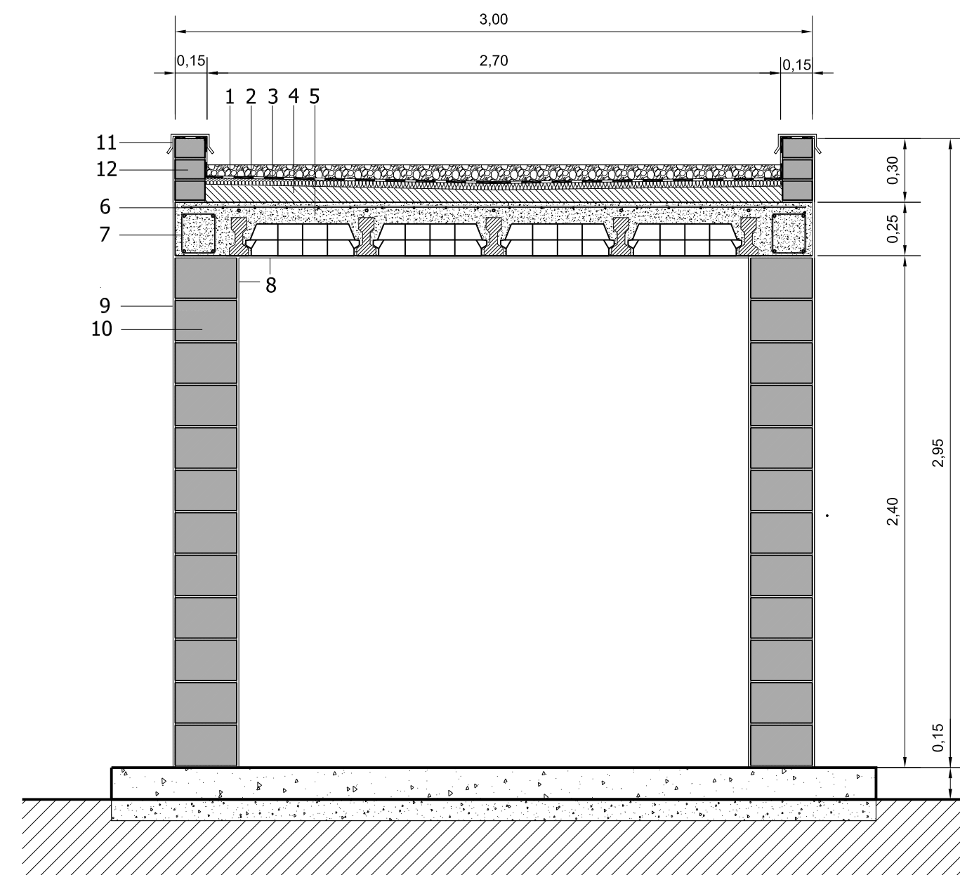
SECCIÓ C-D ESCALA 1/25
