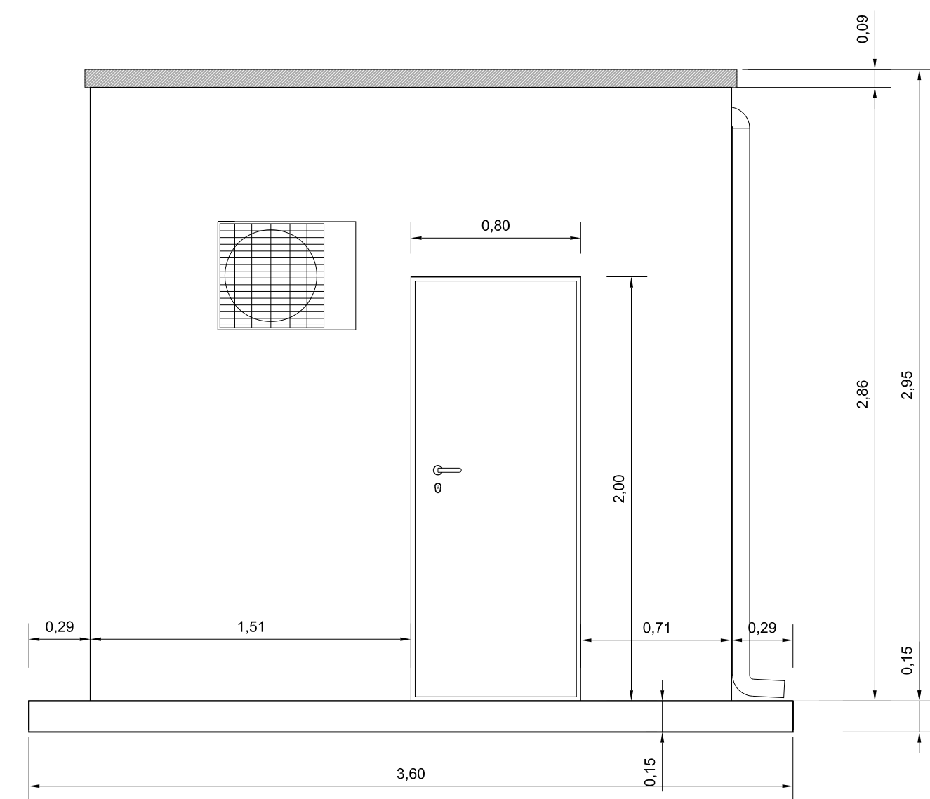
ALÇAT FRONTAL ESCALA 1/25
