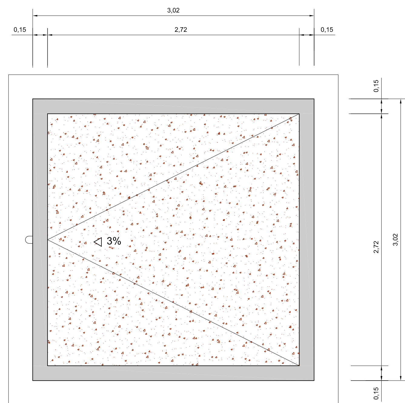
PLANTA COBERTA ESCALA 1/25
