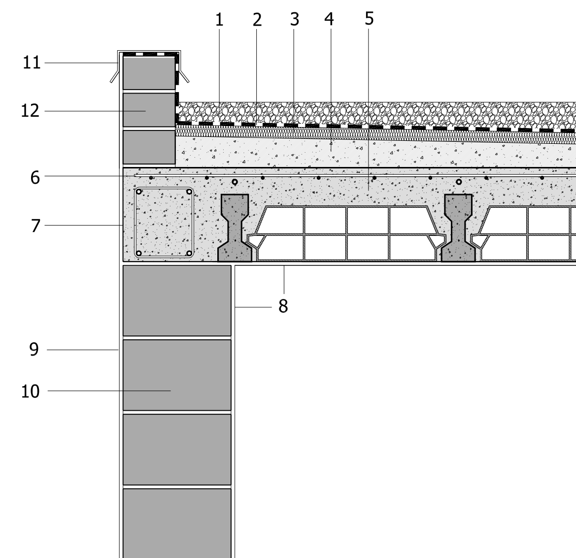
DETALL CONSTRUCTIU COBERTA ESCALA 1/10
