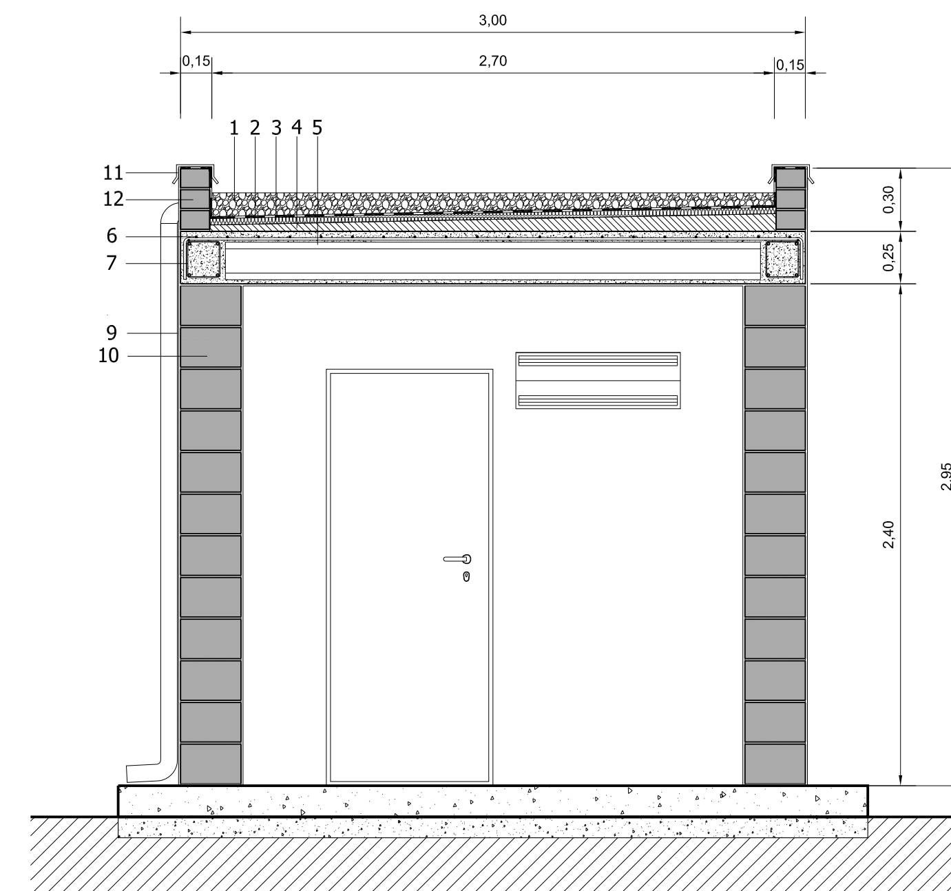
SECCIÓ A-B ESCALA 1/25
