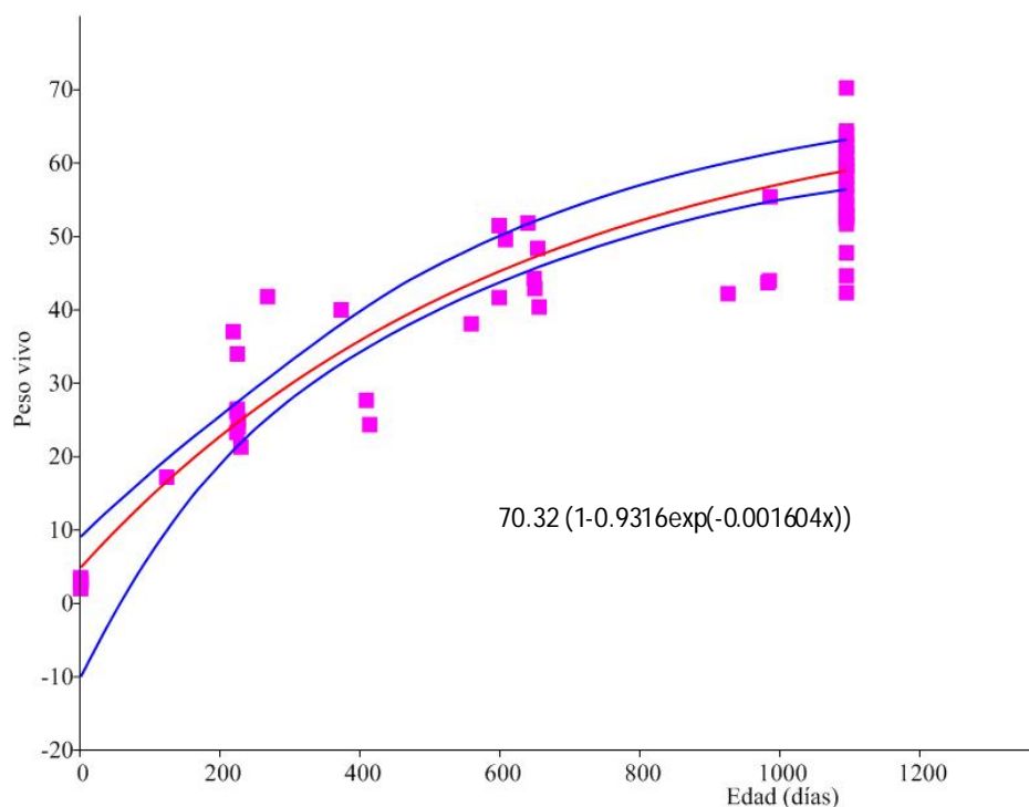
Figura 3. Curvas de crecimiento observadas y predichas para para cabras catalanas hembras (según el modelo de von Bertalanffy) (n=56). Los trazos externos indican el intervalo de confianza del 95%. Peso vivo expresado en kilogramos
