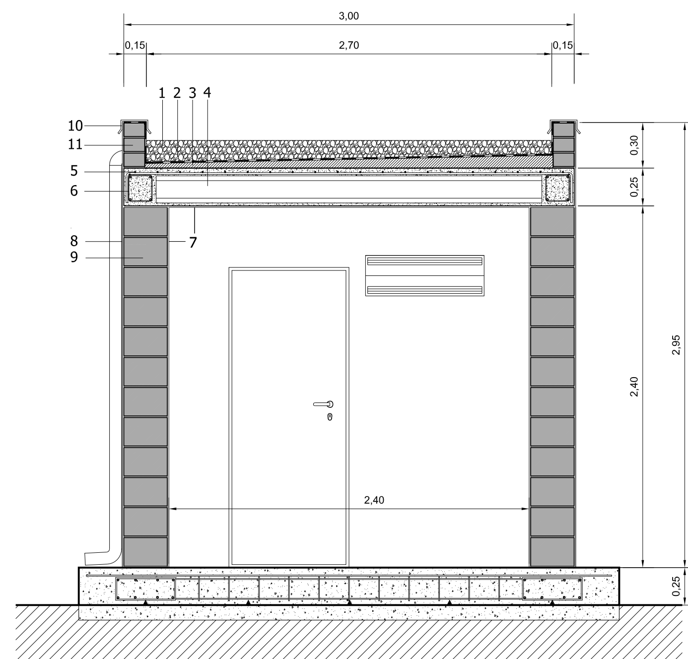
SECCIÓ A-B ESCALA 1/25
