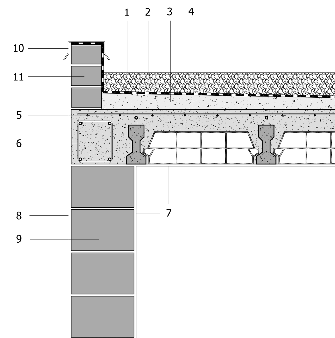
DETALL CONSTRUCTIU COBERTA ESCALA 1/10
