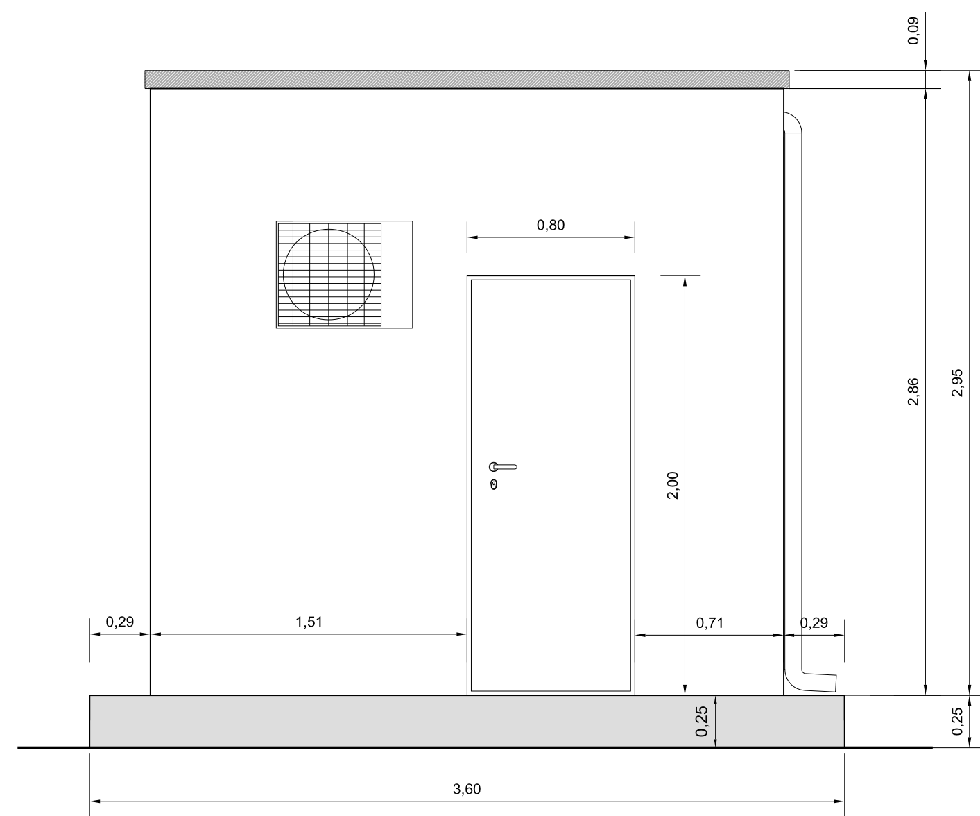
ALÇAT FRONTAL ESCALA 1/25
