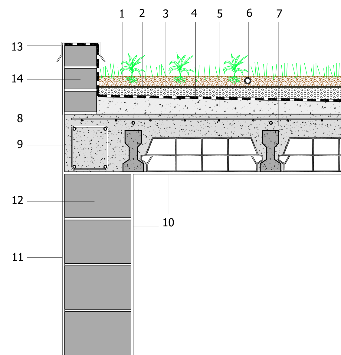
DETALL CONSTRUCTIU COBERTA ESCALA 1/10
