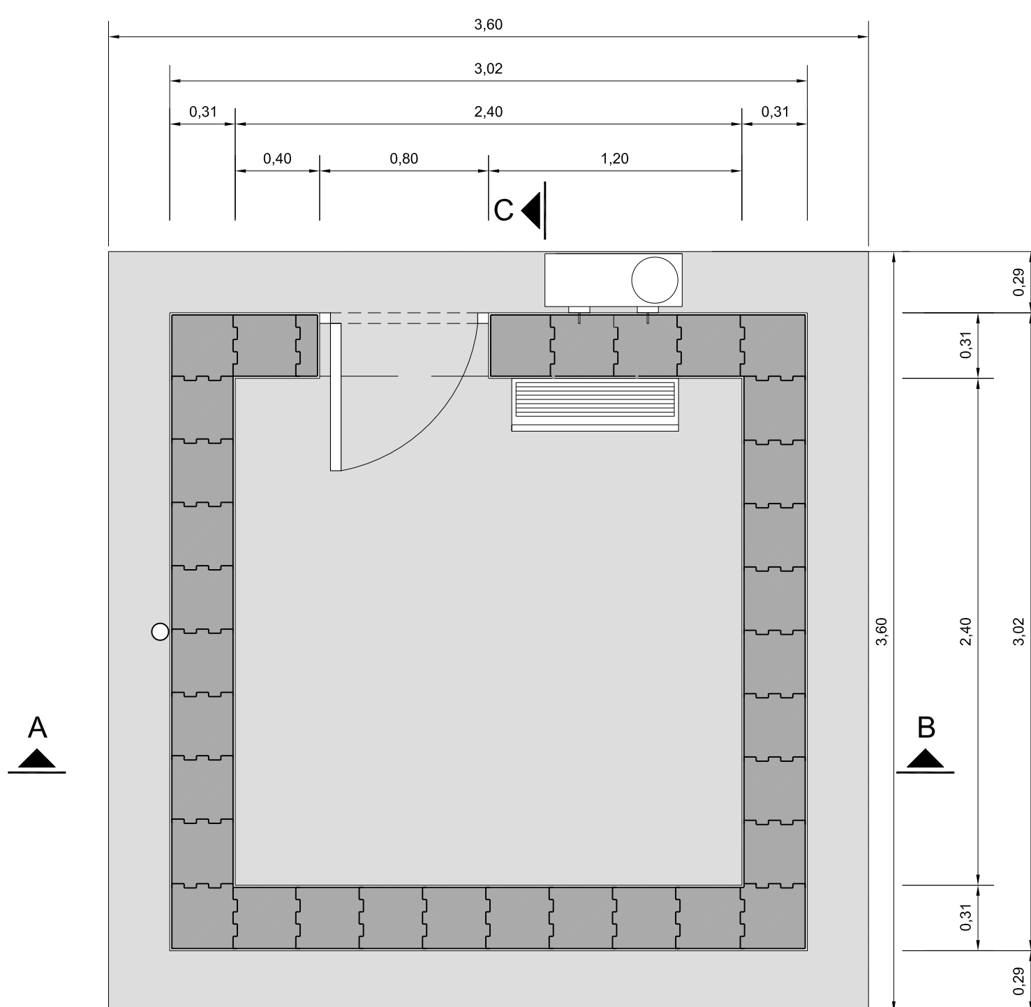
PLANTA ESCALA 1/25
