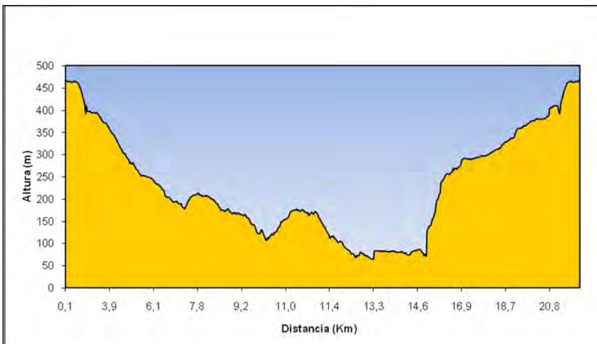
Figura 425: Gràfic altimètric.
