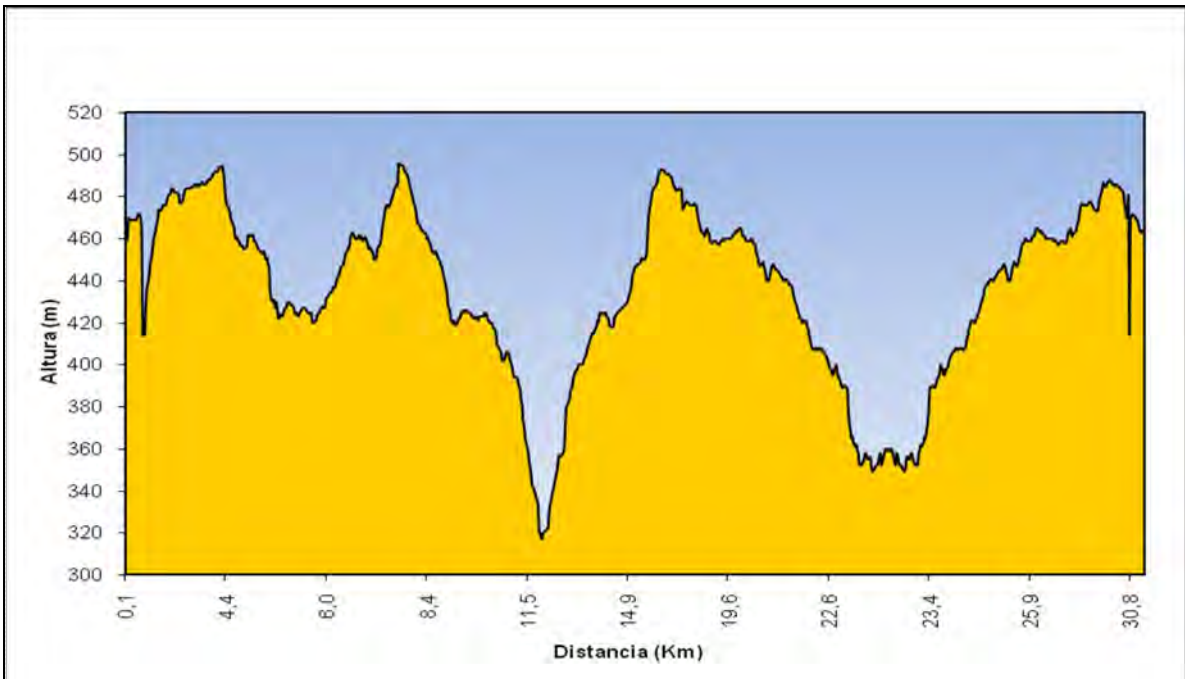
Figura 445: Gràfic altimètric.
