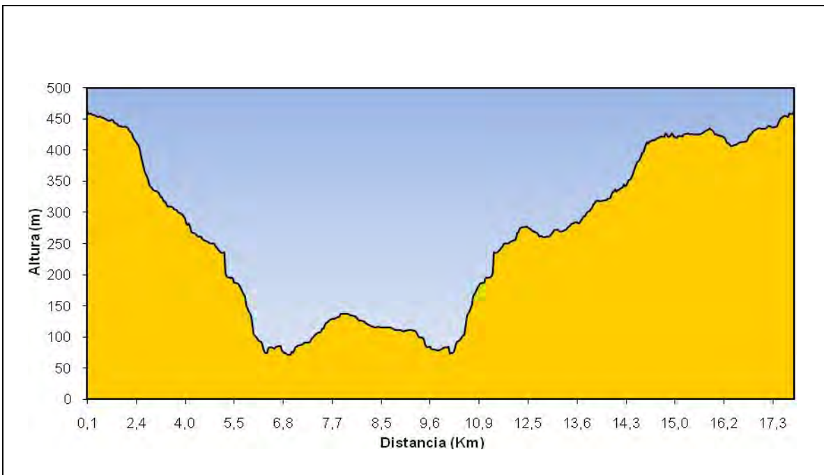
Figura 437: Gràfic altimètric.
