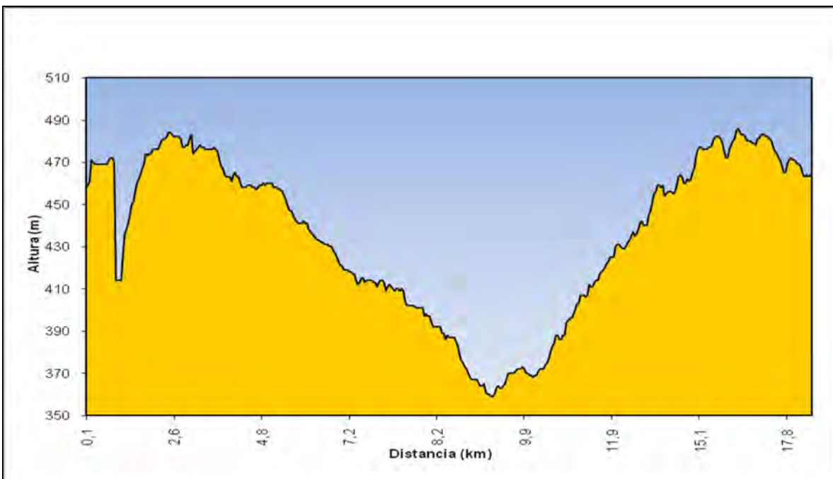
Figura 415: Gràfic altimètric.
