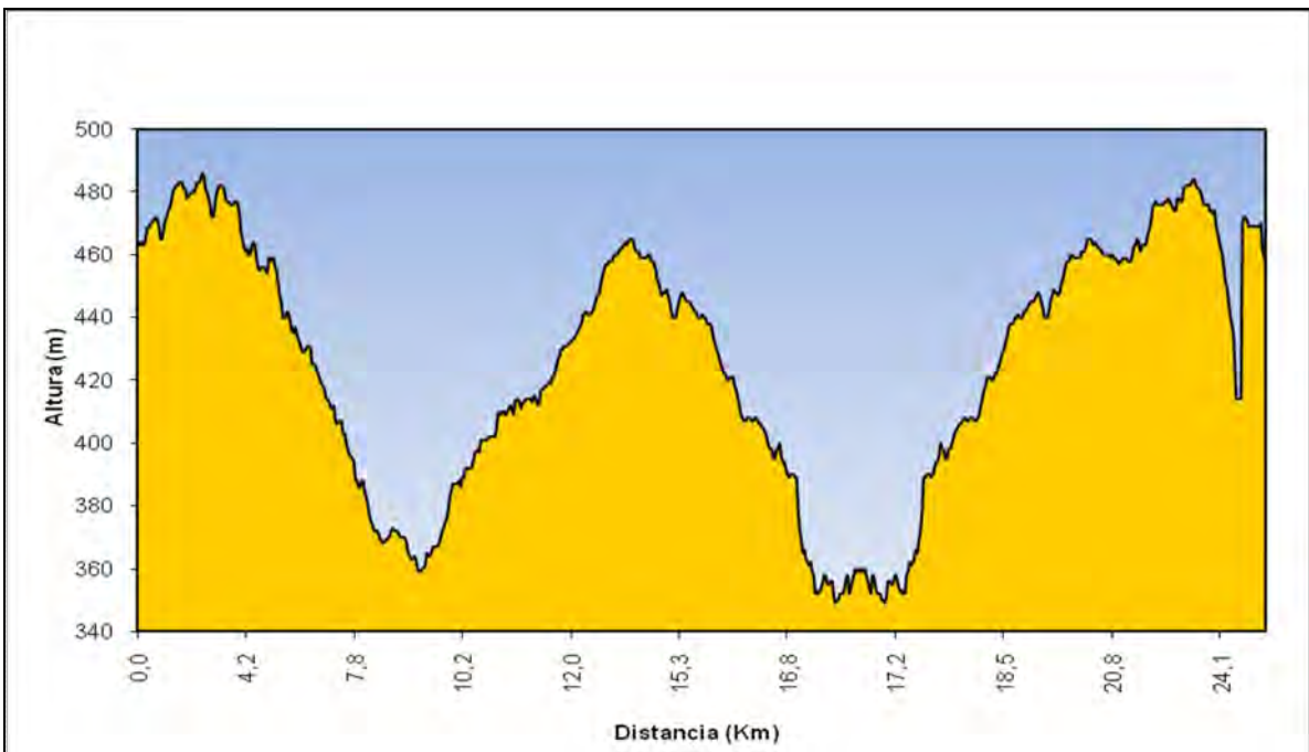
Figura 441: Gràfic altimètric.
