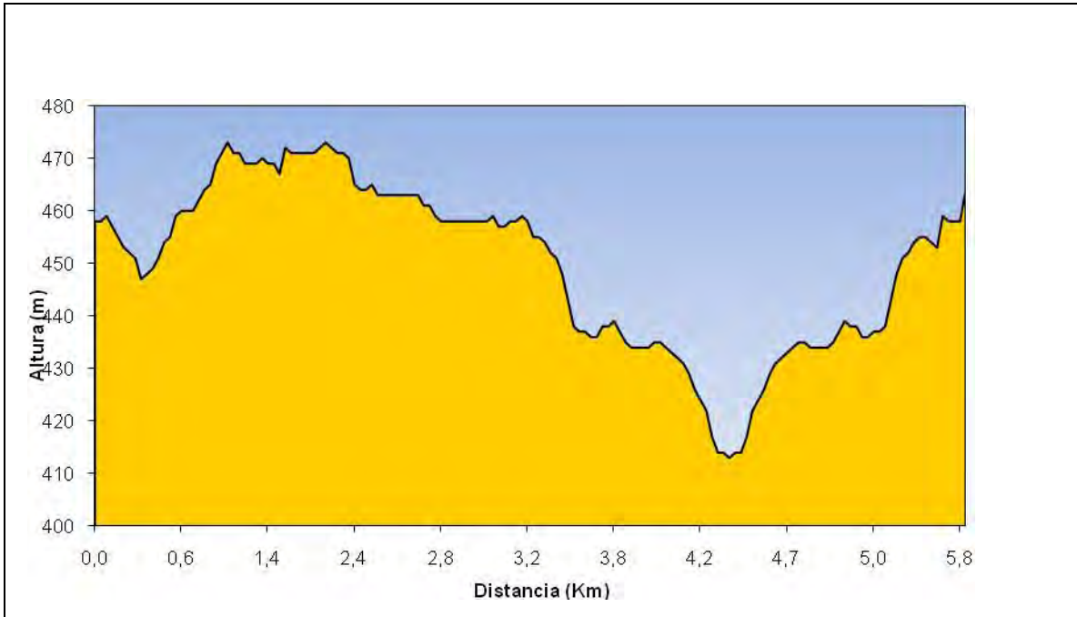
Figura 405: Gràfic altimètric.
