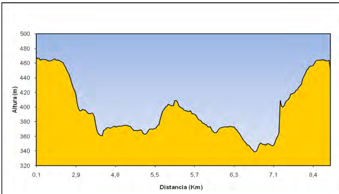
Figura 411: Gràfic altimètric.
