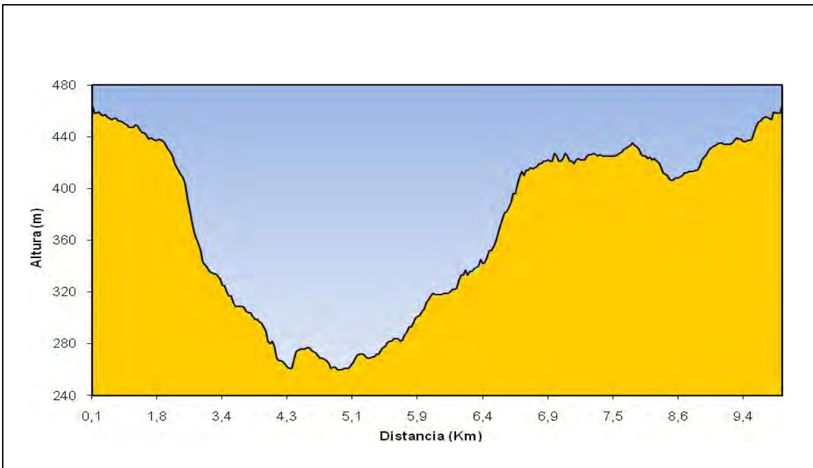
Figura 447: Gràfic altimètric.
