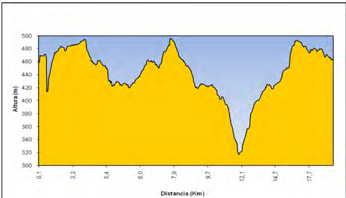
Figura 417: Gràfic altimètric.
