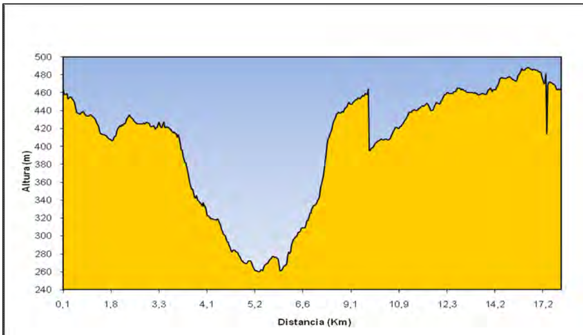
Figura 449: Gràfic altimètric.
