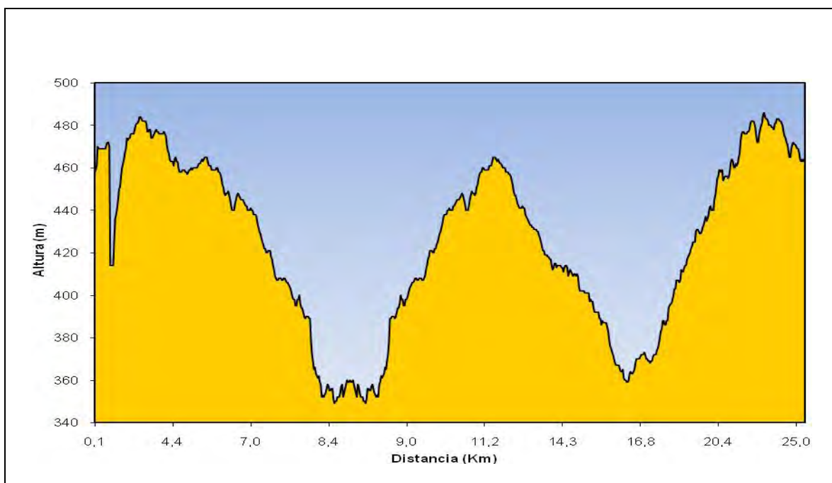
Figura 439: Gràfic altimètric.
