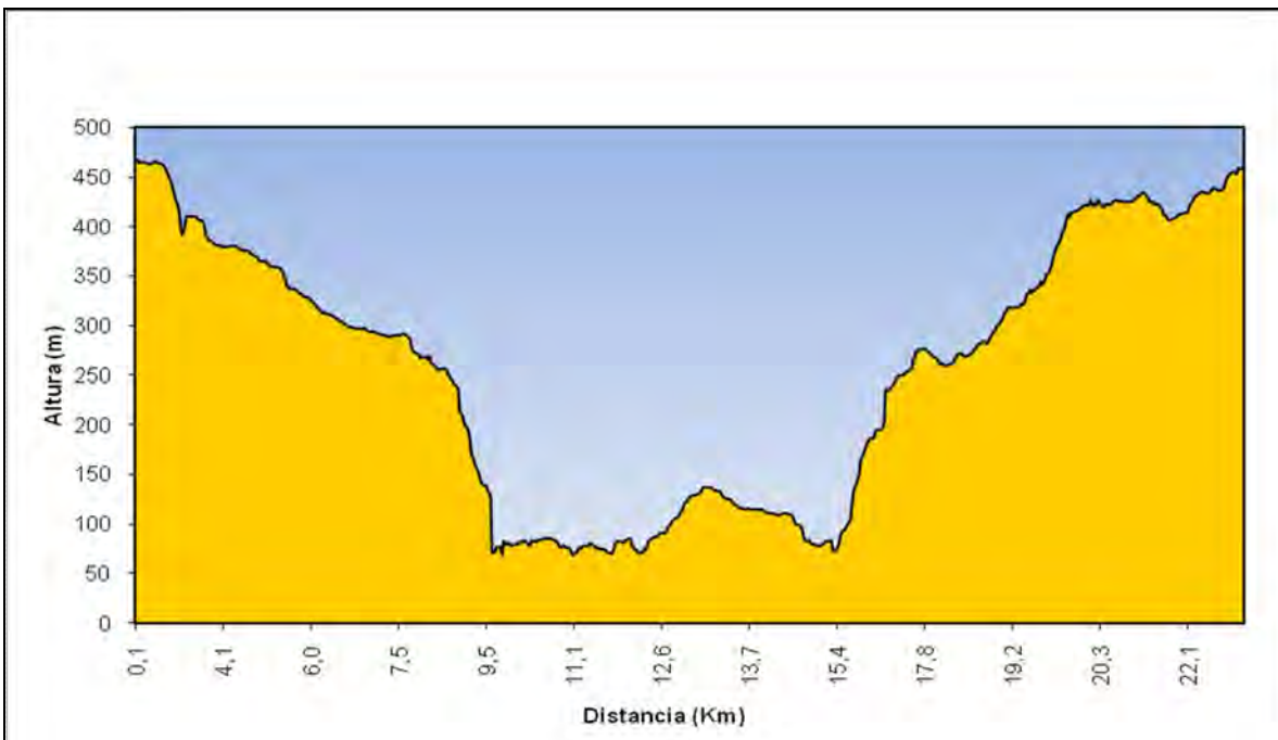
Figura 455: Gràfic altimètric.
