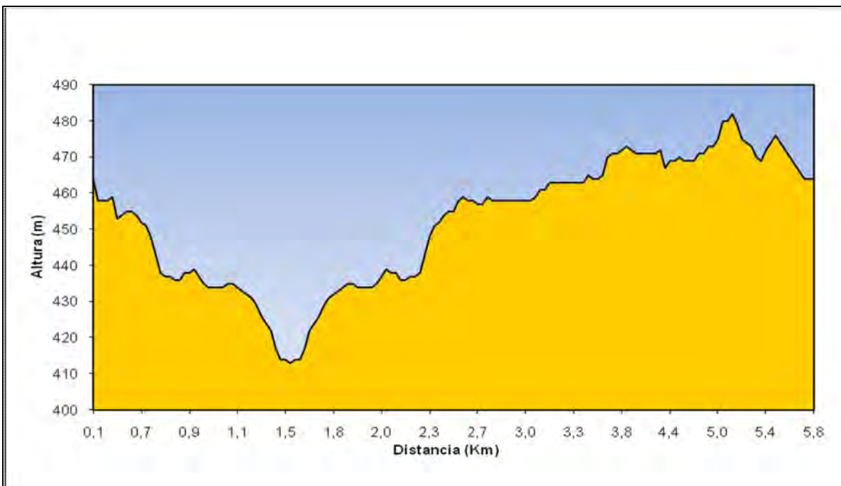
Figura 407: Gràfic altimètric.
