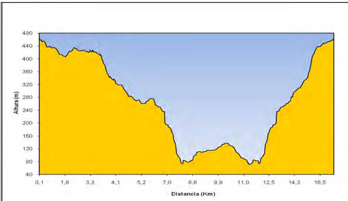
Figura 435: Gràfic altimètric.
