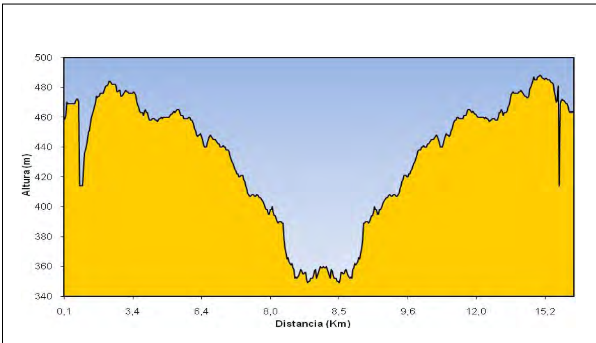
Figura 421: Gràfic altimètric.
