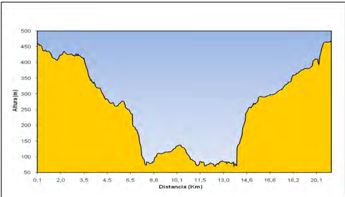
Figura 457: Gràfic altimètric.
